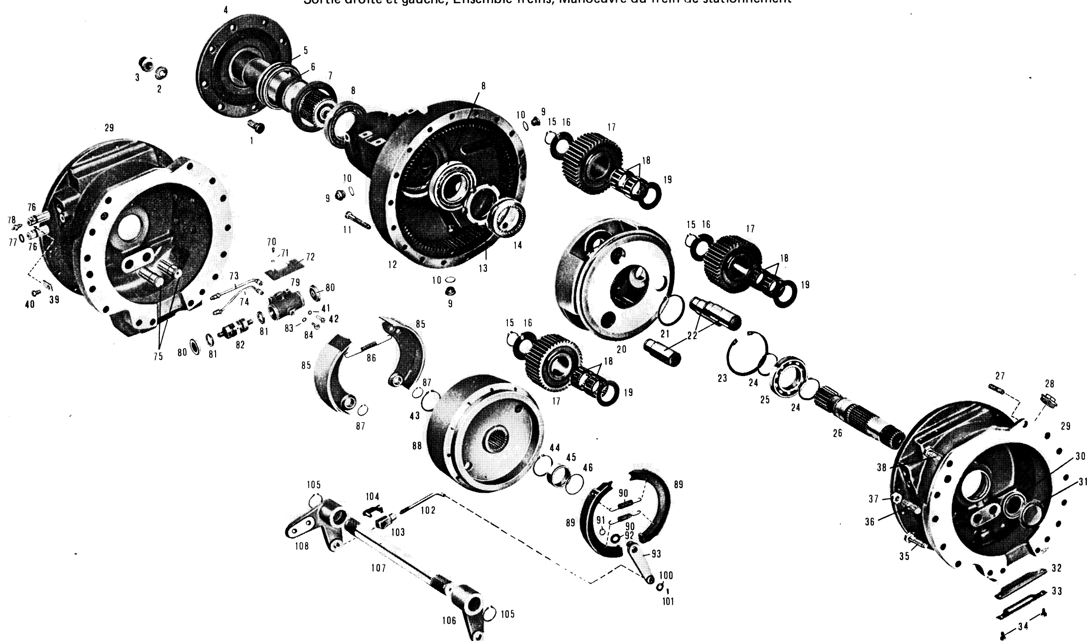
Tafel/Table/Planche 9 T - 3450 Schlüter Abtrieb rechts und links, Bremsen, Feststellbremsbetätigung Final drive RH and LH, Brake assemblies, Parking brake actuation Sortie droite et gauche, Ensemble freins, Manoeuvre du frein de stationnement
