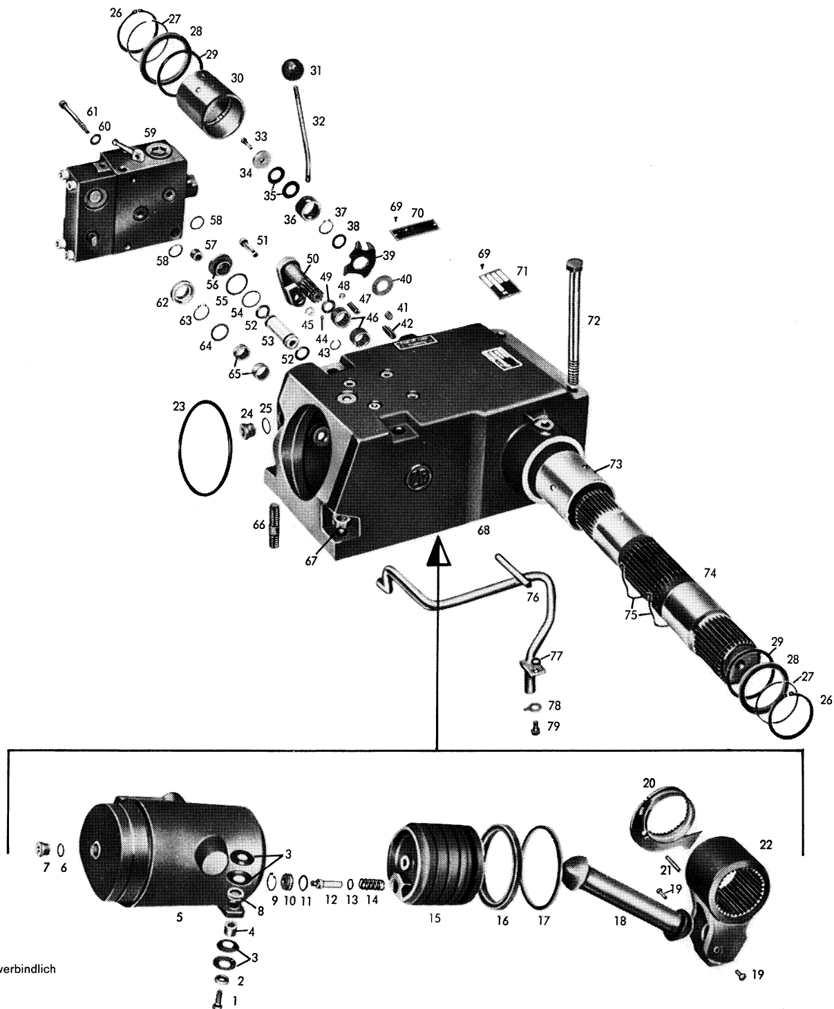
Tafel/Table 7 Regelkraftheber KR - 25 Renault
